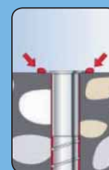
Schroef gelijk met de oppervlakte indraaien, injectiemortel komt naar buiten toe.
