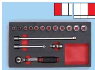
Dopsleutelassortiment 3/8" Metrisch, 16-delig Art. nr. 0965 900 102
