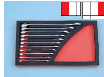
Zebra ringsteeksleutelset Metrisch, 11-delig 15° gebogen ring Art.nr. 0965 900 403
