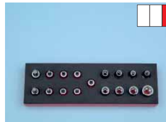
Doppenassortiment 1/2" Binnen- en buitentorx, 17-delig Art.nr. 0965 900 201
