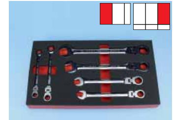
Knieringratelsteeksleutelassortiment Metrisch, 6-delig Met flexibele ringratel Art.nr. 0965 900 410
