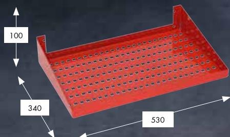
Schap t.b.v. adapterplaat
