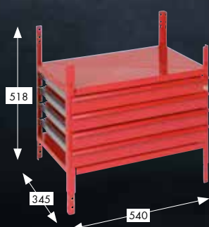
Ladengedeelte, 4 laden
