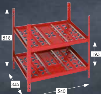
Schappengedeelte voor Würth kunststof bakken gr. 3
