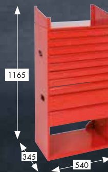
Ladengedeelte, 10 laden
