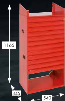
Ladengedeelte, 12 laden
