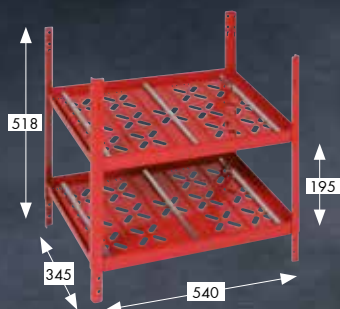
Schappengedeelte voor Würth kunststof bakken gr. 2
