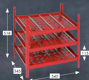
Schappengedeelte voor Würth kunststof bakken gr. 4/5
