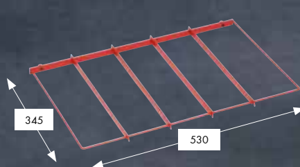
Houder achterlicht
