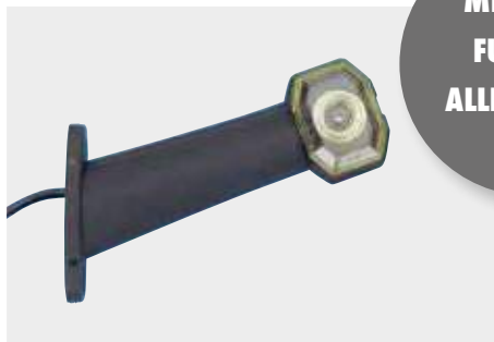
60°-contourlamp Art.nr. 0812 42 203 VE/st. 2
