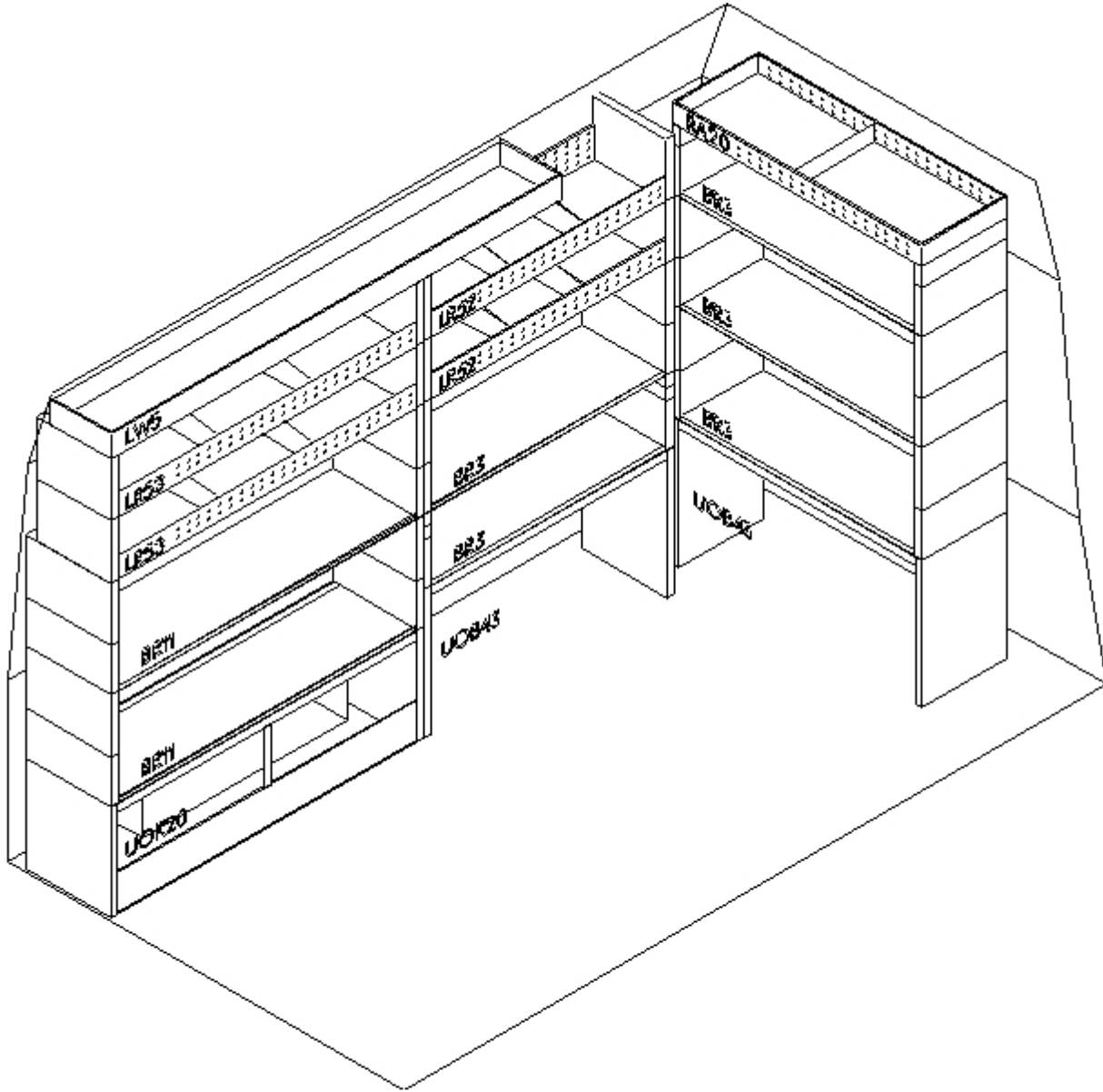
3D-Ansicht, links
