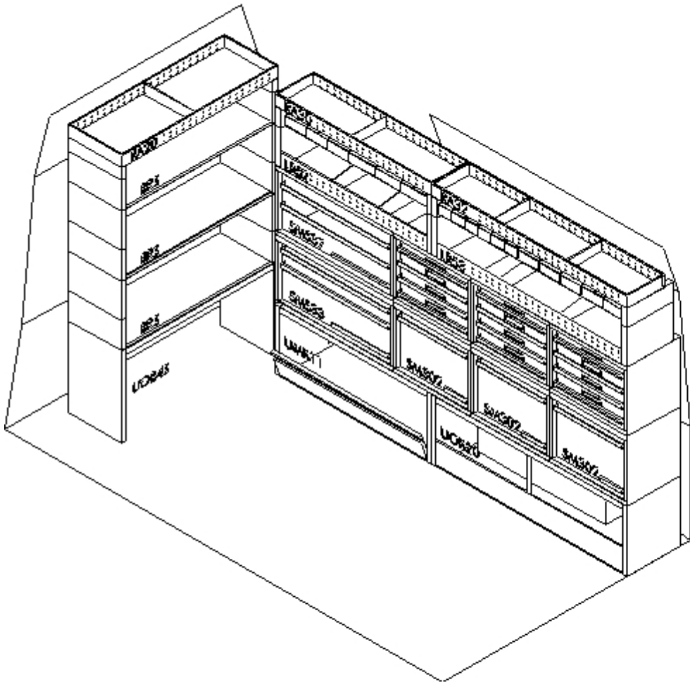
3D-Ansicht, rechts
